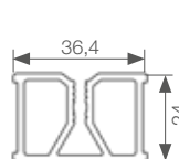
wymiary niskiego legara aluminiowego (mm)
