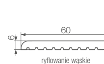
wymiary kompozytowej listwy wykończeniowej (mm)
